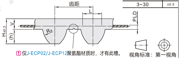
经济型 ECP01-S2M (齿距: 2)
