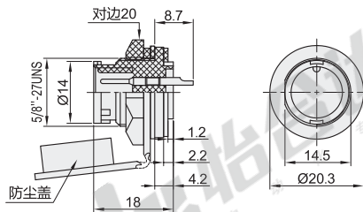
面板安装公插座 ZIX74
