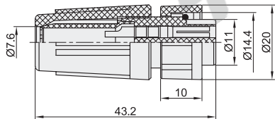
面板安装公插座 ZIX74
