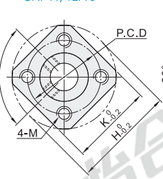
方法兰型 GAF11/12/16
