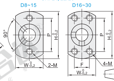
对边法兰型 GAF21/22/26
