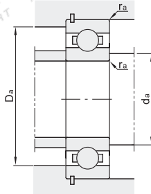
安装图
