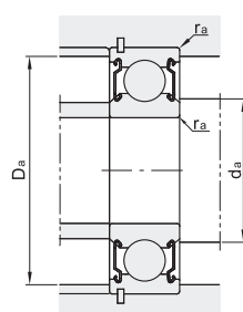
安装图
