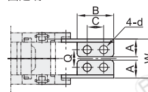
固定端
