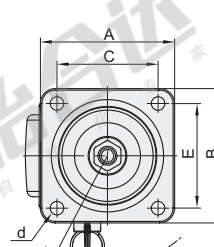
安装面 D60/75
