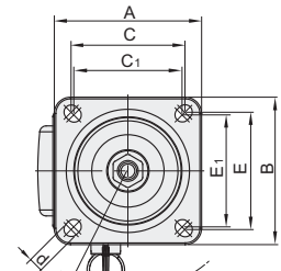
安装面 D60A/75A
