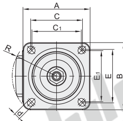
安装面 D60A/75A
