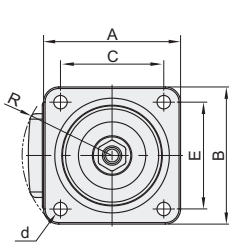
安装面 D60/75
