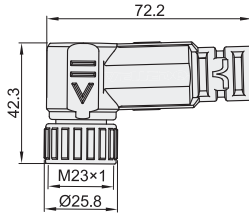
弯母头
