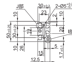
型材截面放大图
