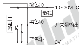
NPN输出
