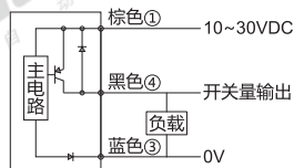
PNP输出
