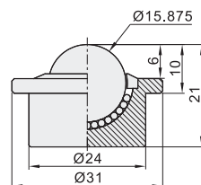
重型 QDB06/07-15
