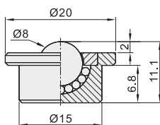
重型 QDB06/07-8
