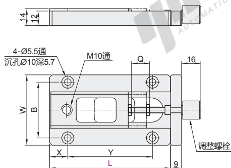
拉力型 ZCL50/51
