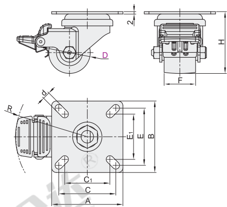
V型孔(塑料单刹) J-CVB36
