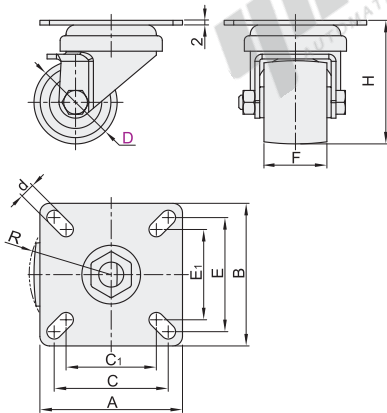
V型孔(无刹) J-CVB35
