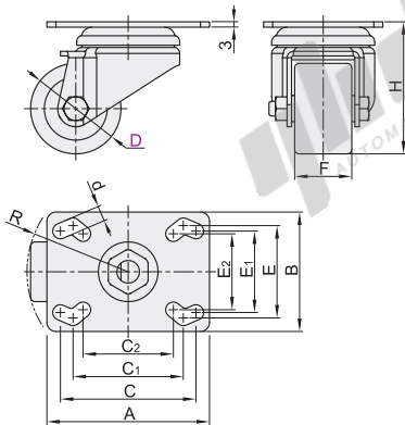
V型孔(无刹) J-CVB35
