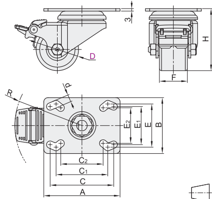
V型孔(塑料单刹) J-CVB36
