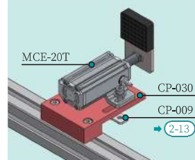
安装例 MCE-20T+CP-030+CP-009
