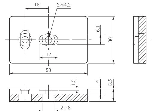
垫板·方形·白2孔· 微型气缸用
