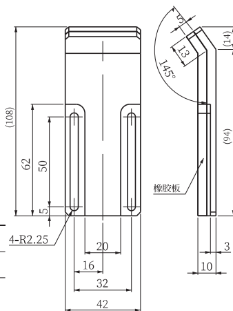
垫板·微型用
