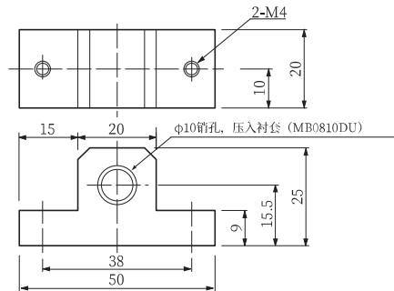
滑移板·微型气缸用
