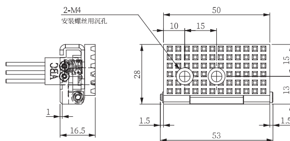
垫板·方形·带白色SW·微型气缸用
