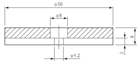
垫板·圆形·白φ50· 微型气缸用
