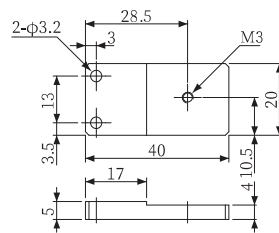
垫板・平行夹具用
