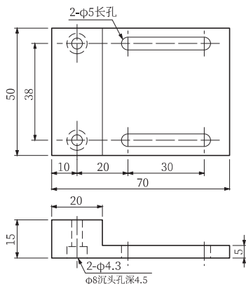
安装例 MCE-20T+CP-030+CP-009
