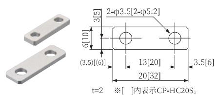
垫板・平行夹具用
