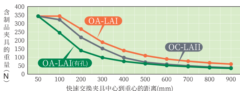
OA-LAI (有孔)、OA-LAI、OC-LAII 静态的许容负荷曲线
