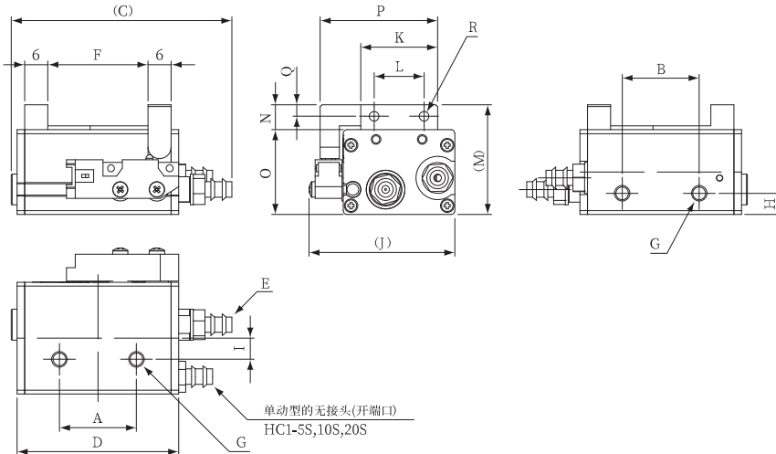
HC1系列外形尺寸
