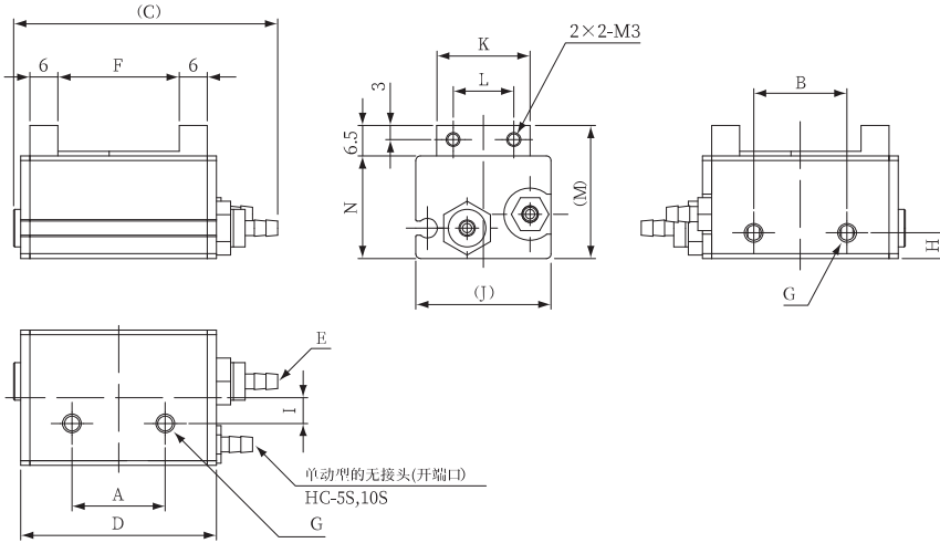
HC1系列外形尺寸
