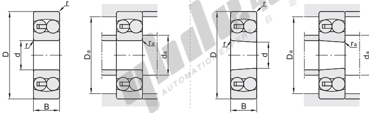
圆柱孔型
