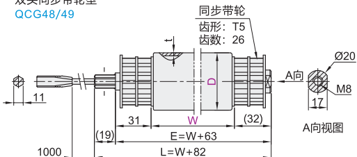
双头同步带轮型 QCG48/49
