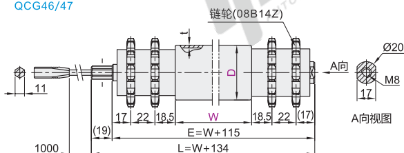
双头双链轮型 QCG46/47
