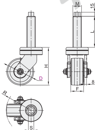
无刹 J-CPM10
