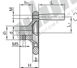
键槽孔型 HAM01 HAL51 螺钉锁紧型 HAL53 方孔型 HAL56
