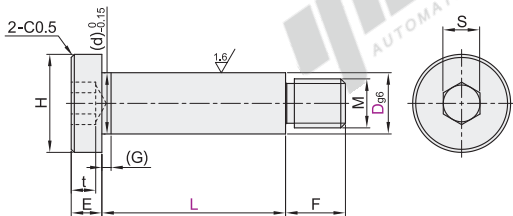
标准型 Y-KCD52/56/58
