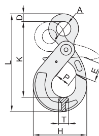
G100眼型安全钩 TCE32
