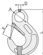
G100眼型滑钩 TCE31
