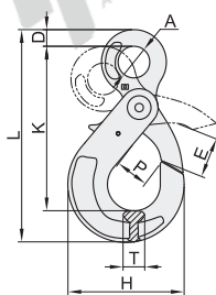
G80眼型安全钩 TCD32
