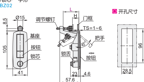
带锁芯·一字形 XBZ02
