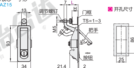
带锁芯·一字形 XA215
