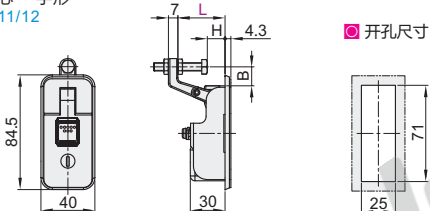
带锁芯·一字形 XA211/12
