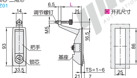
带锁芯·三角形 XBZ01
