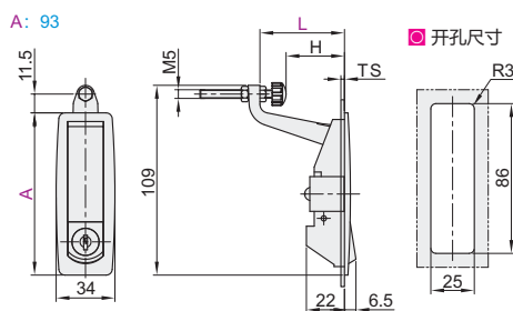
带锁芯·一字形 XA213/14 无锁芯 XA232/33
