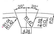
齿形 (ISO标准齿条尺寸)
