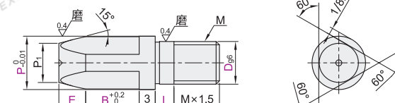
外螺纹型·三角型 YMF51/52/55/56/58
