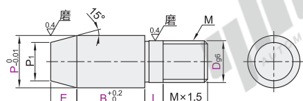
外螺纹型·圆型 YMF41/42/45/46/48
