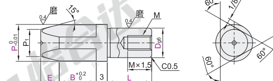
内螺纹型·三角型 YMF31/32/35/36/38
