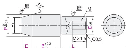
内螺纹型·圆型 YMF21/22/25/26/28
