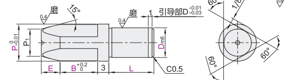
内螺纹型·三角型 YMF31/32/35/36/38
