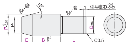
标准型·圆型 YMF01/02/05/06/08
