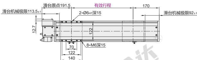
电机安装方式: RD(电机右下折)
