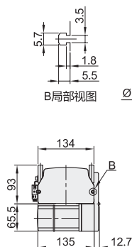
电机安装方式: LD(电机左下折)
