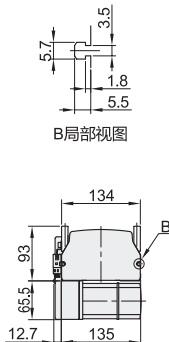
电机安装方式: RD(电机右下折)
