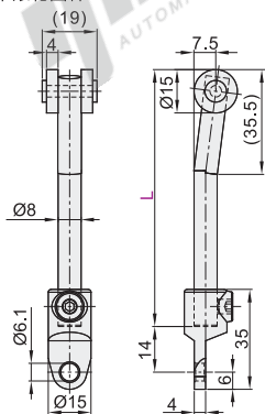
带滚轮圆杆
