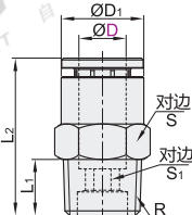
外六角直通接头 XZS42
