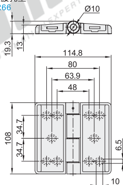
横向腰孔型 HFR66
