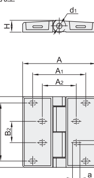
横向腰孔型 HFR67
