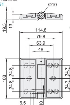
横竖向腰孔型 HFR61
