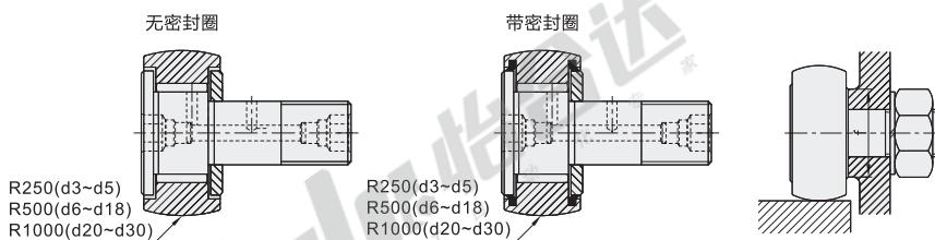
全滚针球面型 E-BPF27/28
