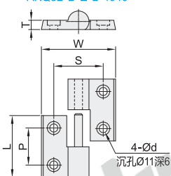
AKQ52-B-Z-L-4040
