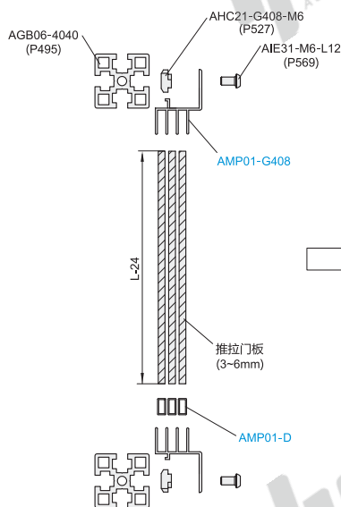
分解图
