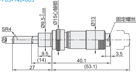
直柄型带心轴锁·球面测量面 EPF03-148-803
