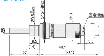
直柄型带心轴锁·平面测量面 EPF03-148-121
