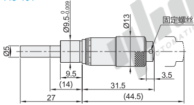
直柄型·平面测量面 EPF03-148-104
