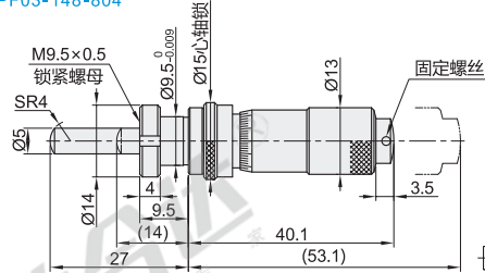
带锁紧螺母·带心轴锁·球面测量面 EPF03-148-804
