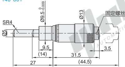
直柄型·球面测量面 EPF03-148-801
