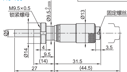
带锁紧螺母·平面测量面 EPF03-148-103
