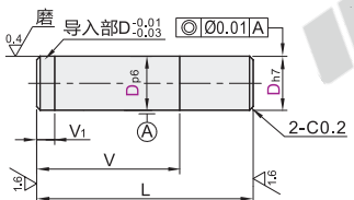
一端p6—端h7 BLX51/52/53
