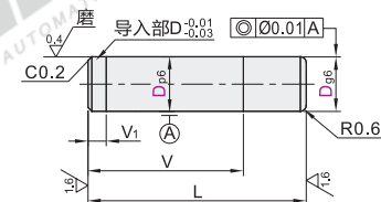
一端p6—端g6 BLX61
