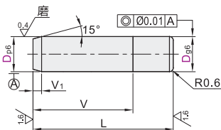
一端p6—端g6 BLX62/63
