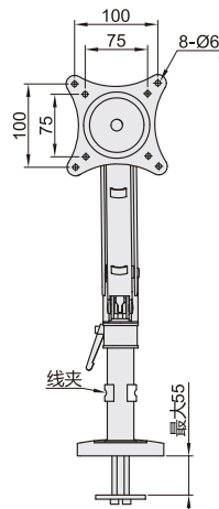
穿孔安装 NHD06
