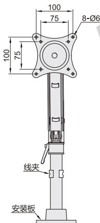
锁孔安装 NHD17
