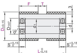
带轴承型 QAJ21
