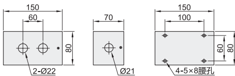
孔数: 2
