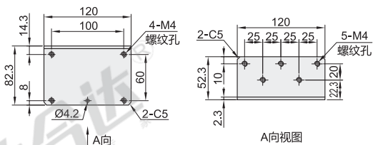
配套支架
