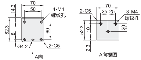
配套支架
