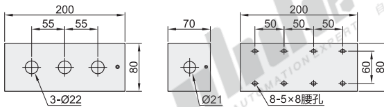
孔数: 3
