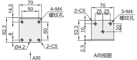
配套支架
