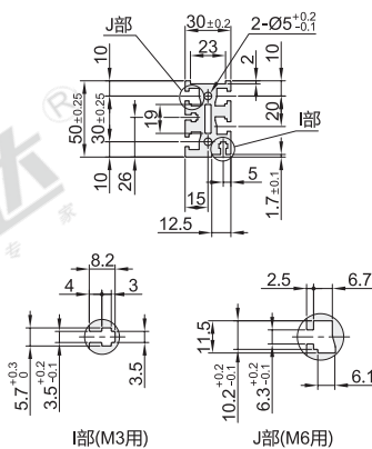
型材截面放大图
