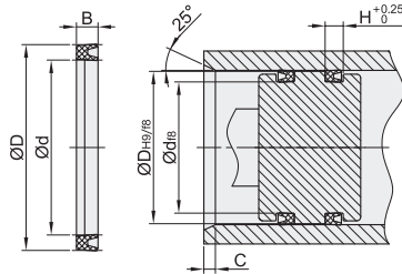
安装尺寸图a
