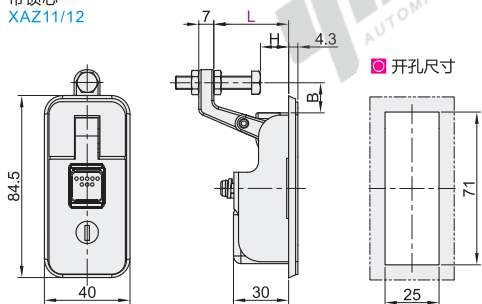
带锁芯 XAZ11/12
