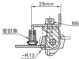
安装尺寸图
