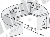
安装尺寸图
