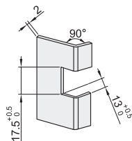
门板开孔
