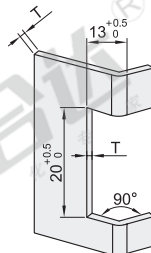
门板开孔
