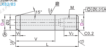
通孔螺纹型 BLX82/83
