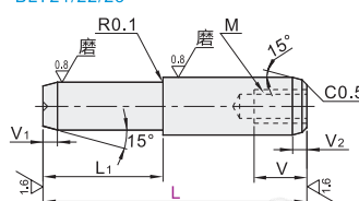
一端内螺纹型 BLY21/22/23
