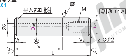
通孔螺纹型 BLX81
