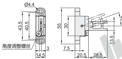
系列: K5 (水平可调整型)
