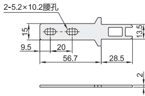
系列: K3 (长T型)
