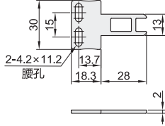
系列: K3 (长T型)
