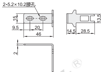
系列: K6 (水平/垂直可调整型)
