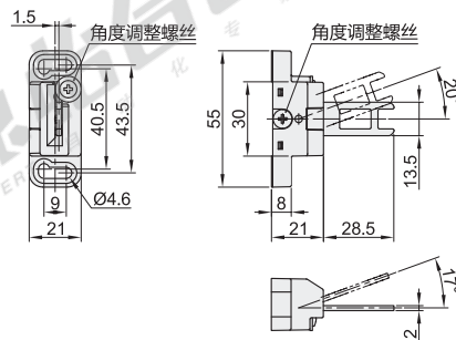
系列: K6 (水平/垂直可调整型)
