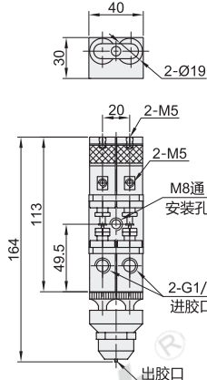
BMD53-04
