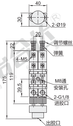
BMD53-06
