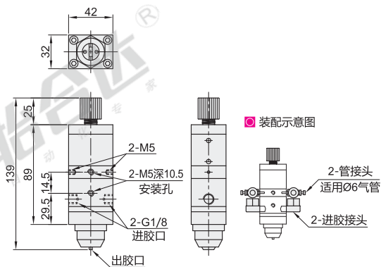
BMD53-10
