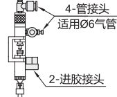
装配示意图
