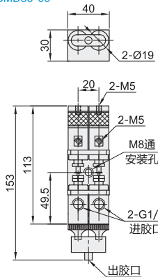
BMD53-03
