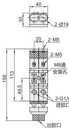
BMD53-03
