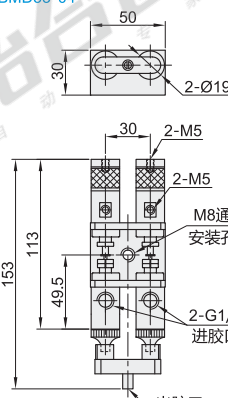
BMD53-04
