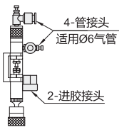
装配示意图
