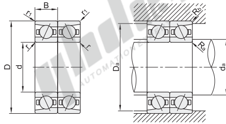
安装图
