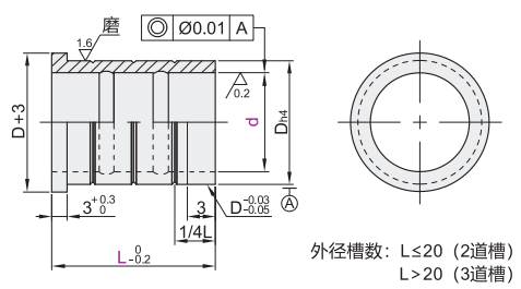
胶粘型·肩型(材质: SUJ2) OFC02
