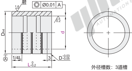
胶粘型·直柱型(材质: SUJ2) OFC01
