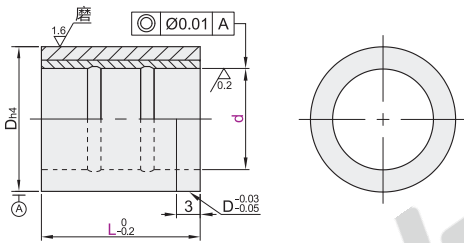
胶粘型·直柱型(材质: SUJ2+铜合金) OFC11
