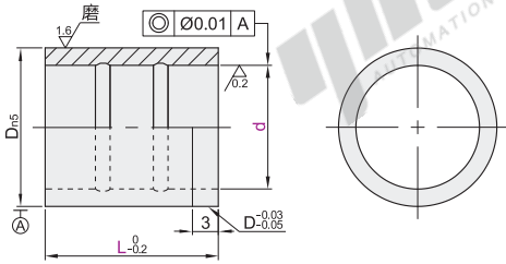
紧配型·直柱型 OFC41
