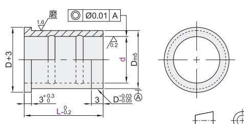
紧配型·肩型 OFC42
