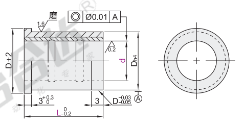
胶粘型·肩型(材质: SUJ2+铜合金) OFC12
