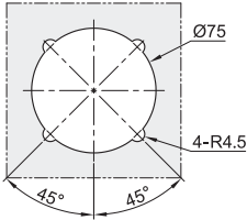
开孔尺寸
