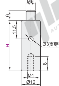
外螺纹型 BMZ27
