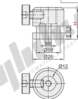
带台阶型 BMZ30
