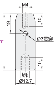
内螺纹型 BMZ26
