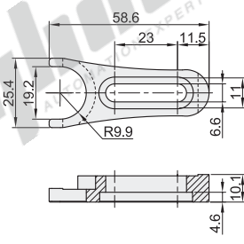
U型 BMZ24
