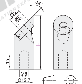
沉孔型 BMZ28
