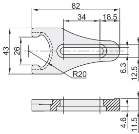
Y型 BMZ23
