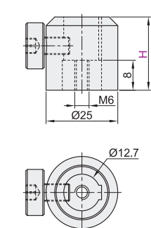
标准型 BMZ29
