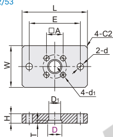
■ 气缸安装形式：螺母安装
