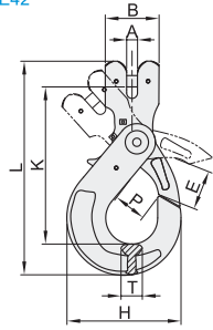
G100羊角安全钩 TCE42
