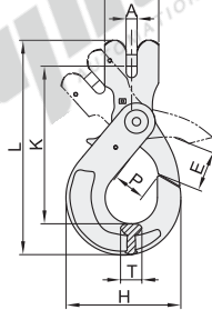
G80羊角安全钩 TCD42
