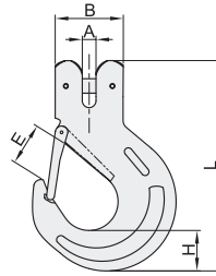
G100羊角滑沟 TCE41
