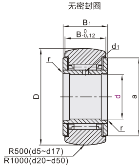
球面型 BPW01/02
