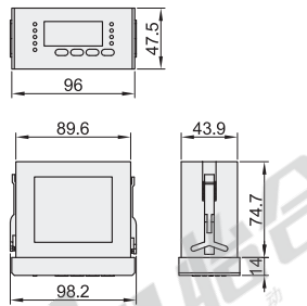
控制器: K2
