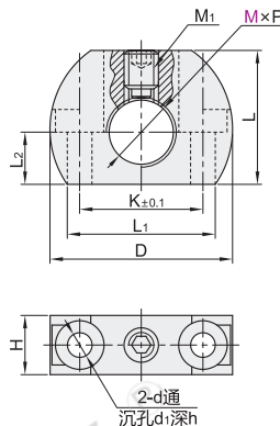
垂直安装型 ZAF65/66
